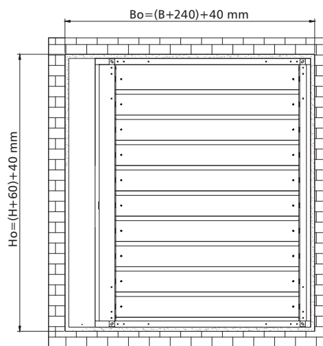
LC - długa obudowa siłownika
