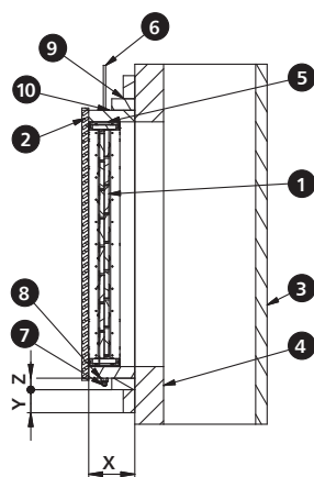
» przekroj pionowy
