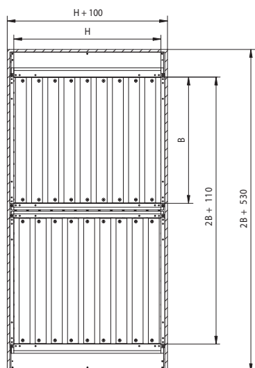
» pionowy
