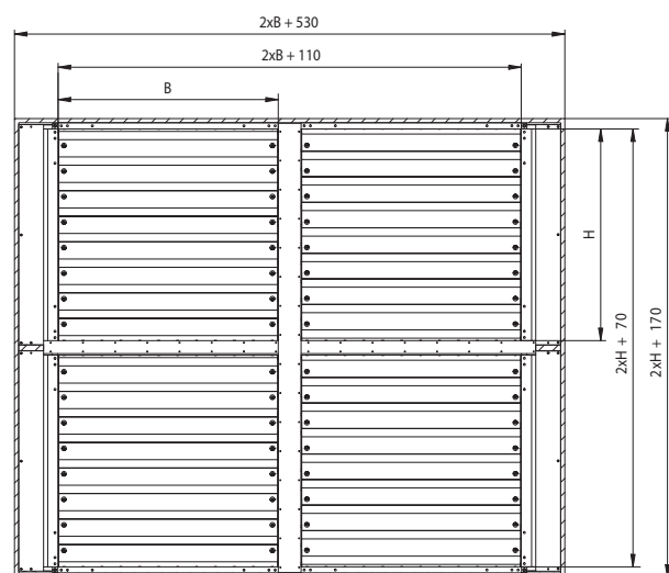
» poziomy
