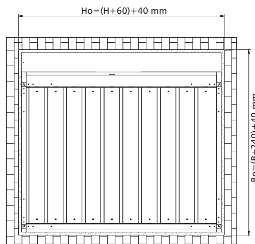
LC - długa obudowa siłownika
