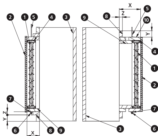
» przekrój pionowy
