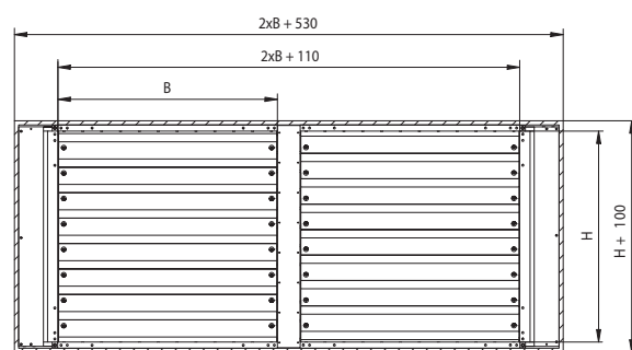
» poziomy
